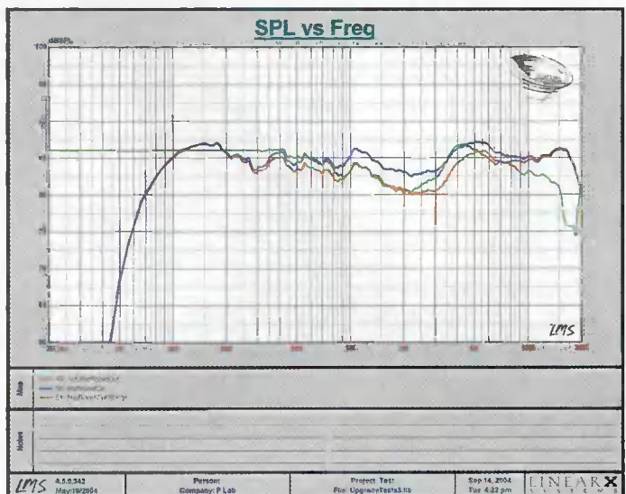
Красная кривая – АЧХ системы на оси, зеленая – под углом тридцать градусов, синяя – снова на оси, со включенной функцией Mid-Boost.
