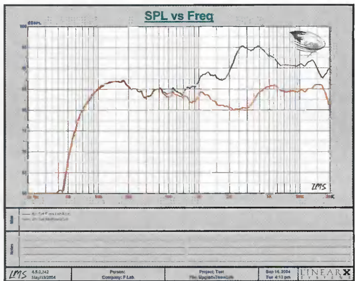
Черная кривая – АЧХ пассивного монитора с лабораторным усилителем, красная – активного монитора (АЧХ корректируется усилителем).
